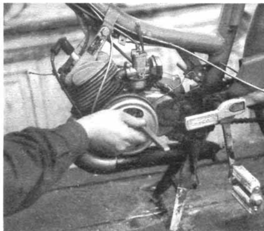
Opération classique : le contrôle de l'écartement des vis platines.
