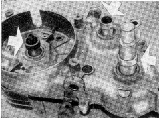
Buchse für Simmerringschutz Ersatzteil 15 Ø = 09.30.34 17 Ø = 09.30.11 20 Ø = 09.30.35
