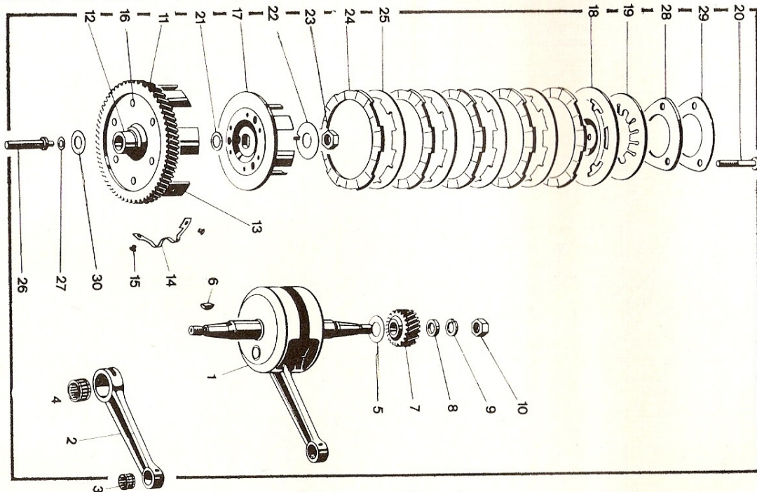
Embrayage et vilebrequin
