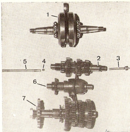
Ensemble mobile du moteur RM 1. Embellage - 2. Arbre primaire - 3. Poussoir du mécanisme de débrayage - 4 et 5. Bille et tige du mécanisme - 6. Tambour de sélection - 7. Arbre secondaire (Photo RMT)
