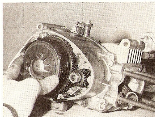
Dépose du ressort à diaphragme et du plateau de pression (Photo RMT)
