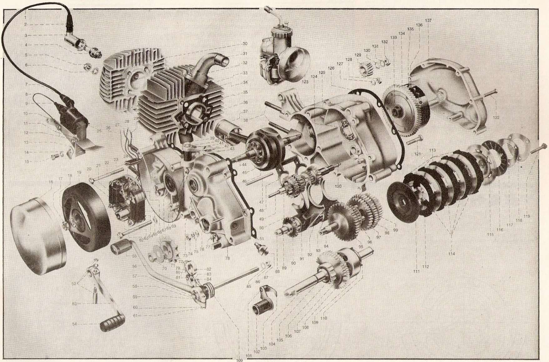
VUE EN ÉCLATÉE DU MOTEUR « RS »
