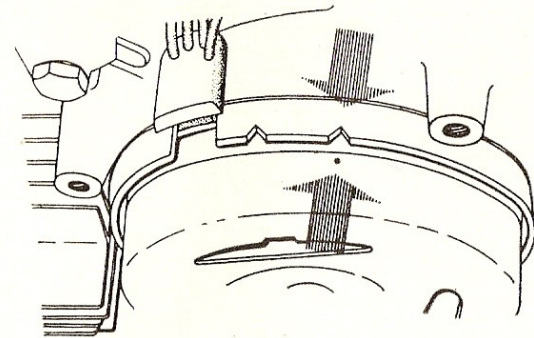
Réglage de l'avance à l'allumage d'après les repères
