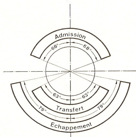
Diagramme de distribution du moteur RM
