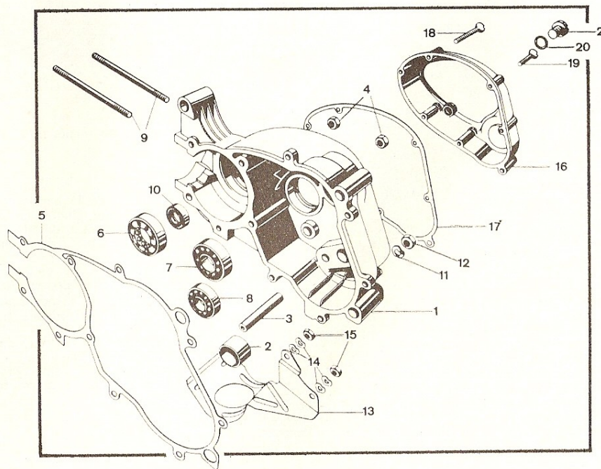
Demi-carter droit et couvercle d'embrayage 1. Demi-carter droit - 5. Joint en papier - 6. Roulement à billes BO 17 DIN 615 - 7. Roulement à billes de l'arbre primaire de boîte de vitesses 6004 C3 - 8. Roulement à billes de l'arbre secondaire 6202 C3 - 9. Goujons de fixation du bloc-cylindres culasse - 10. Joint à lèvre du vilebrequin 17 x 28 x 8 mm - 16 et 17. Couvercle d'embrayage avec son joint - 20-21. Bouchon de remplissage d'huile faisant office de niveau
