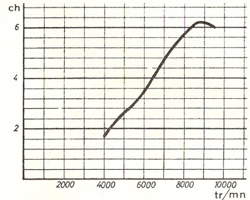
Courbe de puissance du moteur RS
