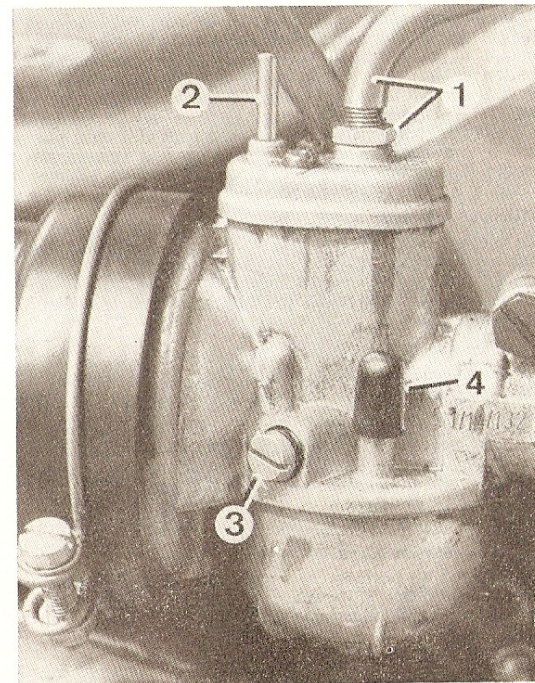
Carburateur du modèle RM
