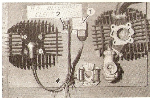
Allumage électronique des nouveaux modèles RS
