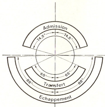
Diagramme de distribution du moteur RS
