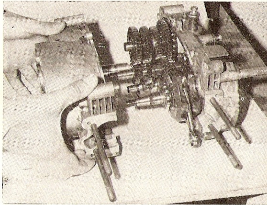
Ouverture des carters-moteurs (Photo RMT)
